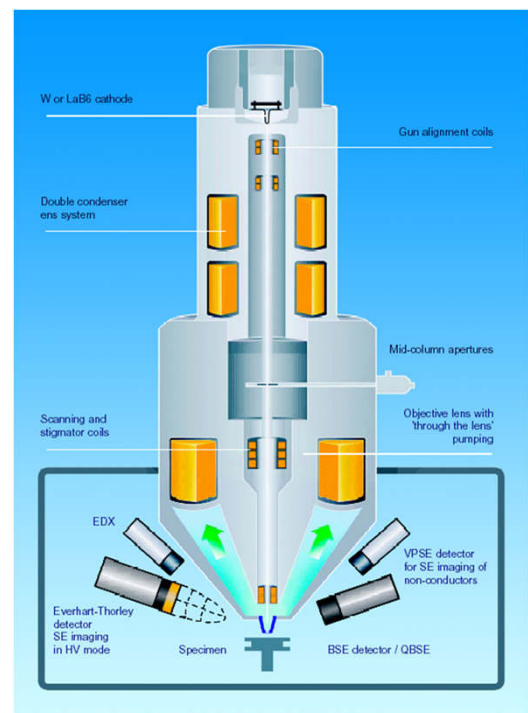
Zeiss: Aufbau EVO-Säule
